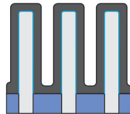
FinFET (FF)
